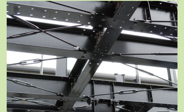
ブレース
