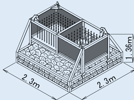
AE-7C型鋼製アオリイカ産卵礁
